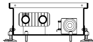
РЕГУЛИРУЕМЫЕ НОЖКИ С КРЕПЛЕНИЕМ К ПОЛУ (ПО ИНДИВИДУАЛЬНОМУ ЗАКАЗУ)
