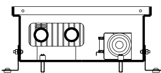
РЕГУЛИРУЕМЫЕ НОЖКИ (БАЗОВАЯ КОМПЛЕКТАЦИЯ)
