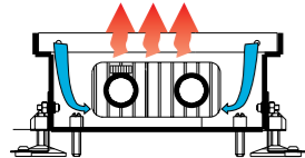
КОНВЕКТОР С ЕСТЕСТВЕННОЙ КОНВЕКЦИЕЙ KE, KEM, KEM1, KEM2
