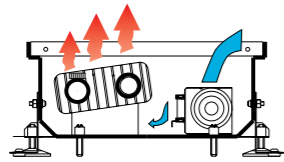
КОНВЕКТОР С ПРИНУДИТЕЛЬНОЙ КОНВЕКЦИЕЙ KV, KVM, KVM2
